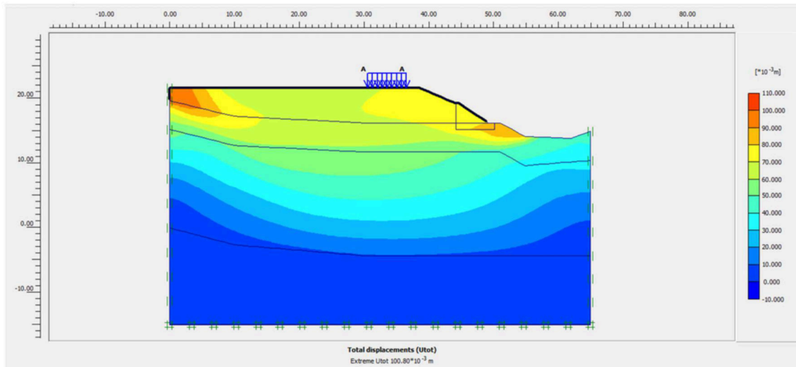
Gambar 3 – Analisa stabilitas DPT kondisi beban gempa dengan SF = 1,14
