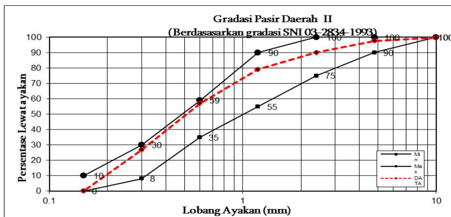
Gambar 7. Hasil Pengujian Analisa Saringan Agregat Halus Desa Dusun Tua Pelang Kecamatan Kelayang
