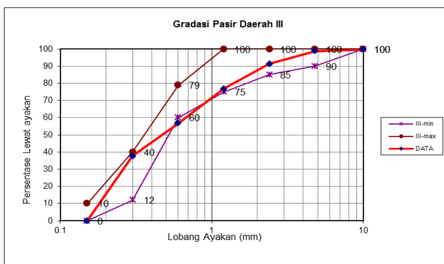
Gambar 5. Hasil Pengujian Analisa Saringan Agregat Halus Desa Pasir Sialang Jaya Kecamatan Lirik
